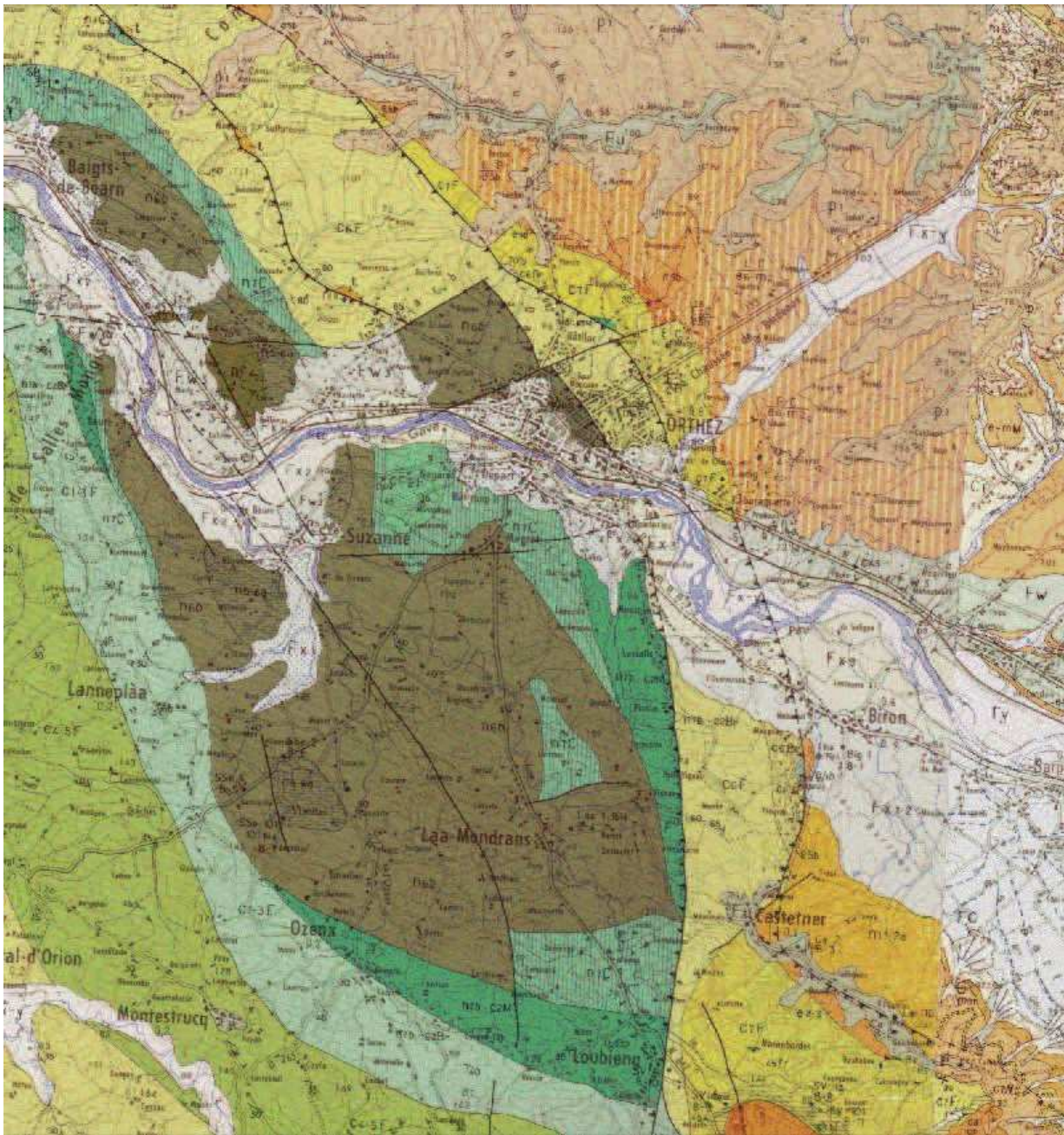
Carte Géologique et matériaux disponibles sur le territoire d'Orthez. Sources : Infoterre BRGM.
