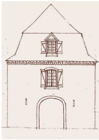
Composition à une travées avec portail : édifice sur trame étroite avec sens de faîtage perpendiculaire à la rue –toit mansardé et croupe sur la rue
