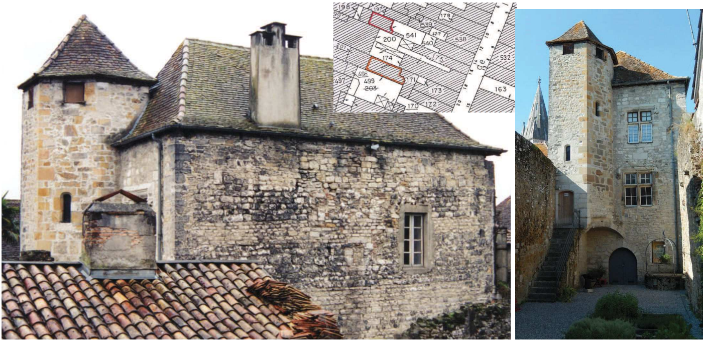
Hôtel de la Lune. Au cœur de l'îlot du Bourg-Neuf, maison fortifiée médiévale remaniée au XV e XVI e siècles. Le corps de bâtiment ancien est constitué de maçonnerie assisée de blocs calcaire (réparée et remaniée). La tourelle d'escalier est ajoutée plus tardivement est constituée de grès jaune issu des carrières de Montalibet. Le rez-de-chaussée est ouvert d'une porte ogivale (XIII e-XIV e), les grandes croisées des baies des étages ont été remaniées plus tardivement (XV e-XVI e).
