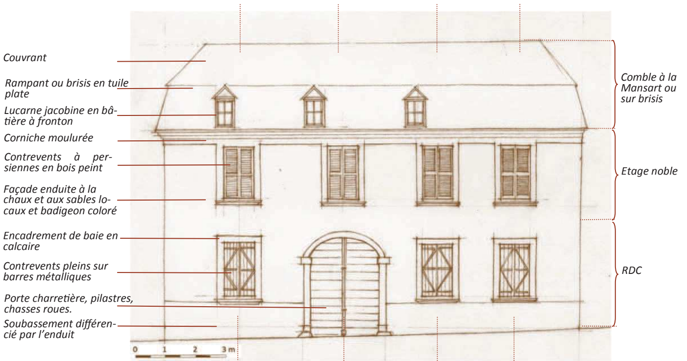
Composition par travées verticales d'ouvertures sur la façade
