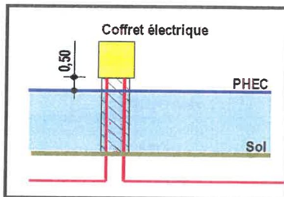
Illustration branchement des habitations
